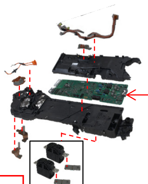
制御ユニット側 部品構成
