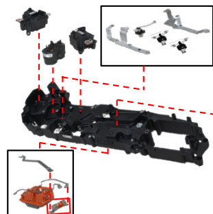
配電ユニット側 部品構成
