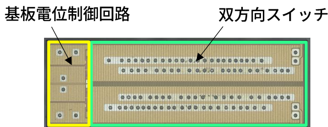
GaN FETチップ
