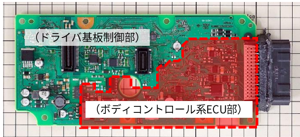
PCU 制御基板 (Bottom view)
